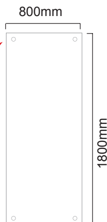
Wymiary grafiki i umiejscowienie przelotek
